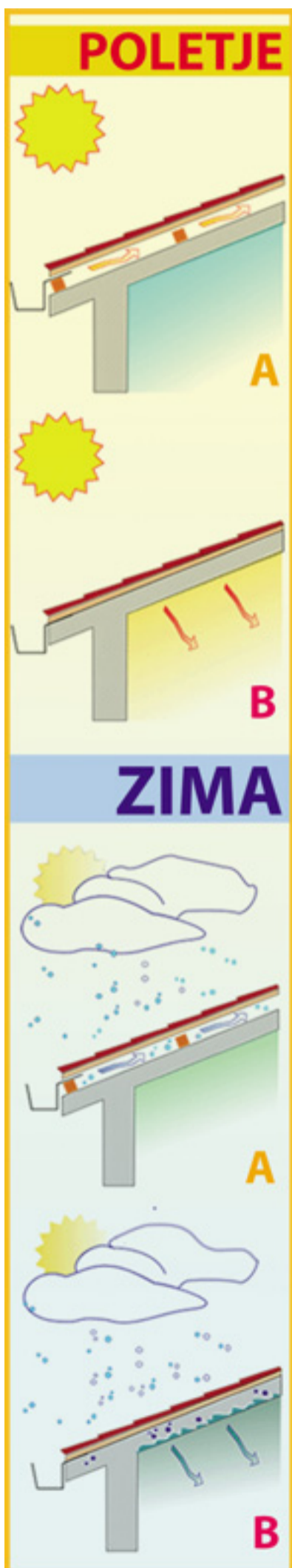
Shema dobro prikazuje prednost prezračevanih streh (A), katerih izolacija je veliko boljše od neprezračevanih (B)
