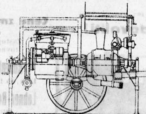
Motorna dvokolna brizgalnica z batnim brzotokim črpalom za visoki pritisk
