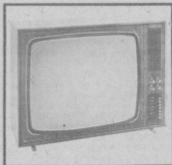
Črno-beli televizor Iskra, PANORAMA ARIES: tiskano vezje, 10 elektronk, 7 tranzistorjev, 21 diod, VHF in UHF kanalnik, ekran 61 cm
