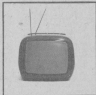
Črno-beli prenosni televizor Iskra Minirama: v sodobni polvodniški tehniki s tranzistorji in integriranimi vezji na tiskani enoti, VHF in UHF kanalnik, priključitev na 220 V ali akumulator 12 V, teža 7,5 kg, ekran 31 cm
