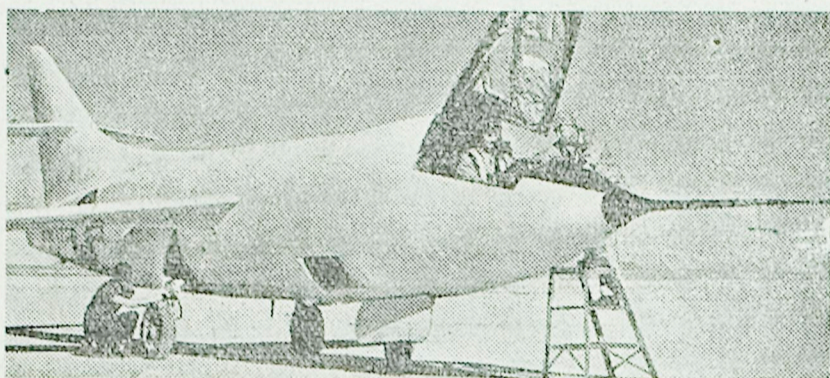
Douglas D 558-2 Skyrocket — tako imenujejo letalo, ki ga vidite na naši sliki. Letalo je na reakcijski pogon in je trenutno najhitreje na svetu. Nov rekord hitrosti sicer še ni potrjen, toda uradno so objavili, da je letalo doseglo skoraj dvojno hitrost zvoka. Znani ameriški poskusni pilot Bill Bridgeman je v višini 25.376 m dosegel z njim hitrost 2.036 kilometrov na uro, kar je skoraj 600 m v sekundi ali 35 km v minuti. Iz Kopa v Ljubljano bi prišli potemtakem s tem letalom v bori 4 minutah! Vsekakor spoštovanja vredna hitrost.
