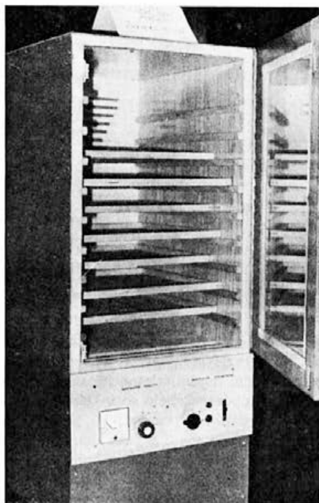
Sušilna naprava za cvetni prah foto: avtor
