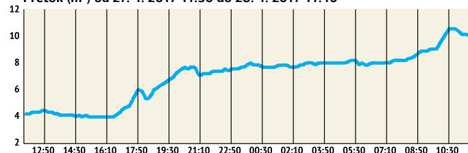
Vodostaj (cm) in pretok Pšate (m 3 /s) na postaji Loka (pri Malnovem mostu, op. a.) med 27. in 28. aprilom 2017 (Vir: ARSO).
