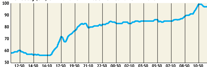
Pretok (m 3 ) od 27. 4. 2017 11:50 do 28. 4. 2017 11:40
