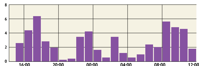
Urna intenziteta 24-urnih padavin (mm) med opoldnevom 27. in 28. aprila 2017. (Vir: Vremenska postaja OŠ Trzin)
