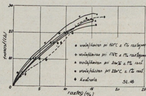
Diagram 17: prikazuje trdnost (razteznost) odnos za vroče fiksiran kord z 1 % raztegom pri temperaturi 150—220°C z dodatnim 20 minutnim nenapetim izpostavljanjem temperature 150°C.
