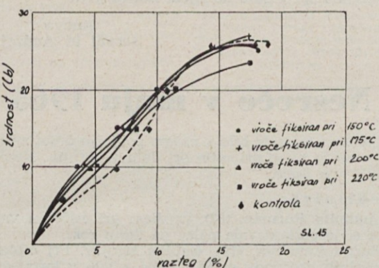
Diagram 15 in 16: prikazujeta trdnost (razteznost) odnos pri katerem po 20 min. fiksiranja pri 150°, 175°, 200° in 225°C z napenjanjem oz. z 1 % raztegom.
