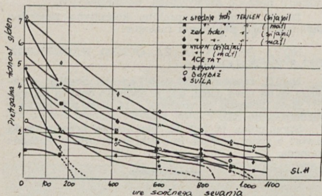
Diagram 11: izguba trdnosti terylena in drugih vlaken zaradi vremenskih vplivov.
