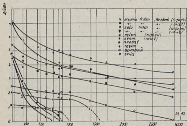
Diagram 12: izguba trdnosti zaradi vpliva sončne svetlobe.
