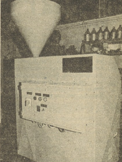
Eden izmed briketerjev, kakršnega so izdelali v TOZD Sestavnih deli in delovna sredstva DO Avtomatika tudi za Polprevodnike v Trbovljah.
