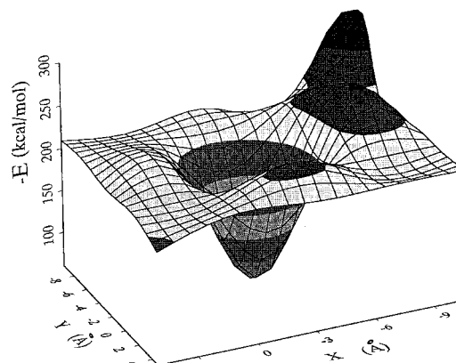
Slika 5a: Površina potencialnih energij za model "aa" Figure 5a: Potential energy surfaces for model "aa"
