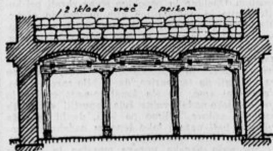
Ojačitev stropa obokane kleti, ki bo služila za zaklonišče.
