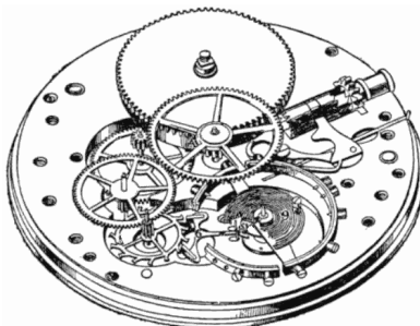
sestavljena ura
