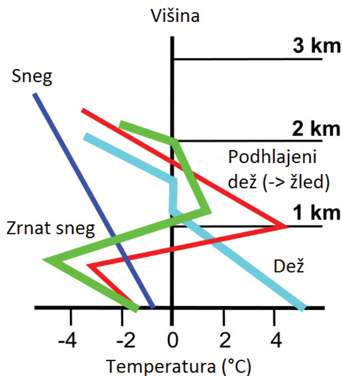
Temperaturni poteki z višino, ki privedejo do različnih vrst padavin
