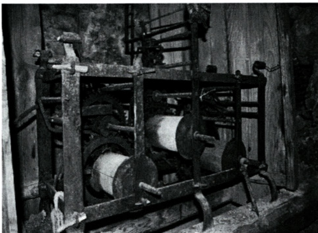
Mehanizem ure v zvoniku (vse foto: R. Brus)
