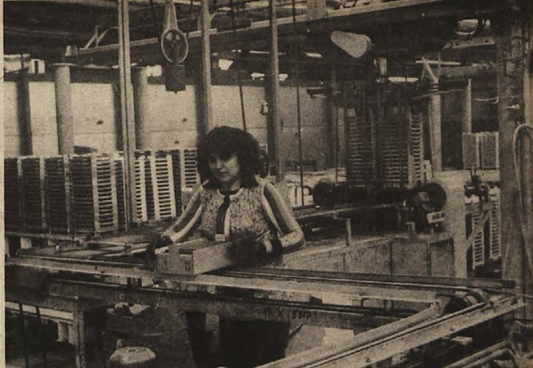
PREPOČASEN STROJ — Prebiralna linija je v Industriji gradbene keramike na Račjem selu ugotovljeno ozko grlo proizvodnje. Predvidena je zamenjava. Ob boljši organizaciji prodaje po novem ne bi smelo biti več težav. (Foto: Železnik)
