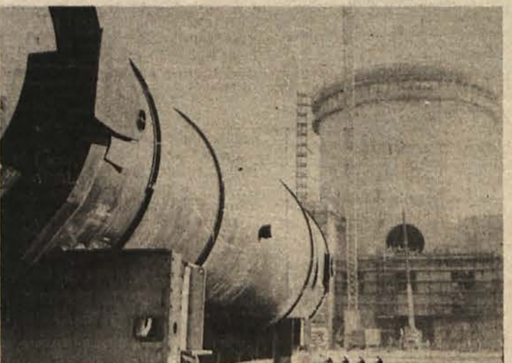
PARNI GENERATOR NA CILJU. Delavcem mariborske Hidromontaže je ta tristo dvajsettonski tovor povzročil ogromno skrbi. Prvega so prepeljali z Reke brez nezgode, drugi pa je za nekaj časa obležal za cesto pri Zgornjem Jelenju. Zdaj je tudi ta skrb mimo. (Foto: Jožica Teppey)
