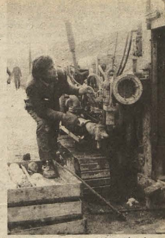
SONDIRANJE - Na kandijski avtobusni postaji pri odcepu ceste h KREMENU Geološki zavod iz Ljubljane že nekaj dni pridno sondira zemljišče in zbira vzorce za geološko analizo sestave tal. To so nujna dela za gradnjo novega cestnega podvoza bodoče cestne obvoznice Brod - Partizanska cesta. (Foto: Koncilija)
