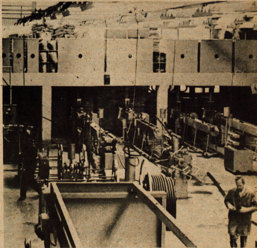
IPI — proizvodnja alkatnih cevi za vodo
