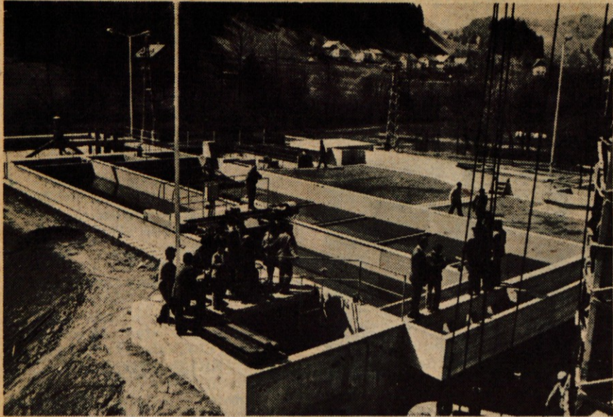
Obsežen kompleks betonskih pretočnih kanalov, zapornic in jaškov tvori jedro mehansko-biološke čistilne naprave na Suhi. Ločani so vanjo investirali skoraj pol milijarde starih din. Če bo poslej Sora res spet takšna kot je bila nekoč, potem se je splačalo, pravijo.
