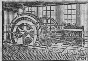
LANZEV ventilni lokomobil za vroči sopar z naravnost prijetim dinamom.
