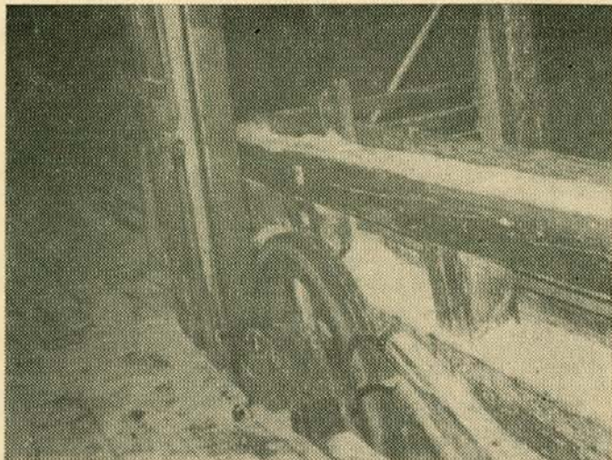
Voz s podajalnim mehanizmom — Mravljakova žaga ob Vuhreščici
