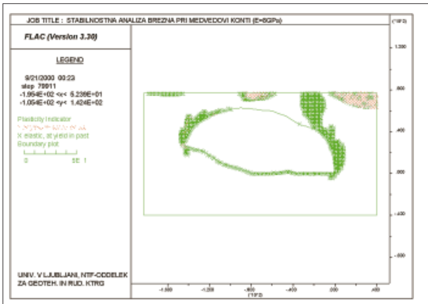
Fig. 4: Plasticity indicators in the surroundings of hall area (ceiling thinner than 20 m). Sl. 4: Plastična območja v hribini v okolici dvorane (strop tanjši kot 20 m).
