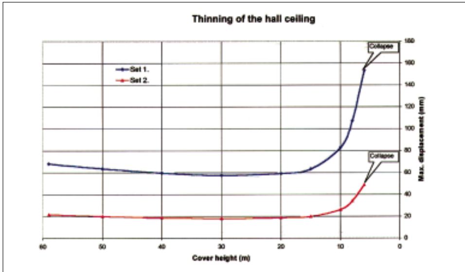
Fig. 3: Thinning of the Medvedova konta hall ceiling. Sl. 3: Tanjšanje stropa dvorane Medvedove konte.
