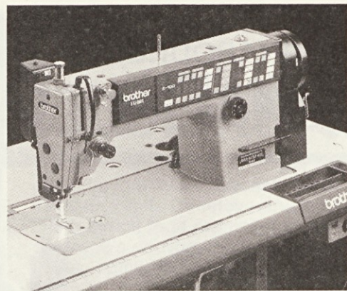
Vsestransko uporabljeni šivalni procesorsko vodeni stroj BROTHER Exedra 737, japonske izdelave.
