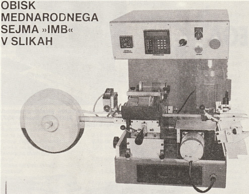
Tiskarski stroj za rezanje in tiskanje tekstilnih etiket S-E/12 L.
