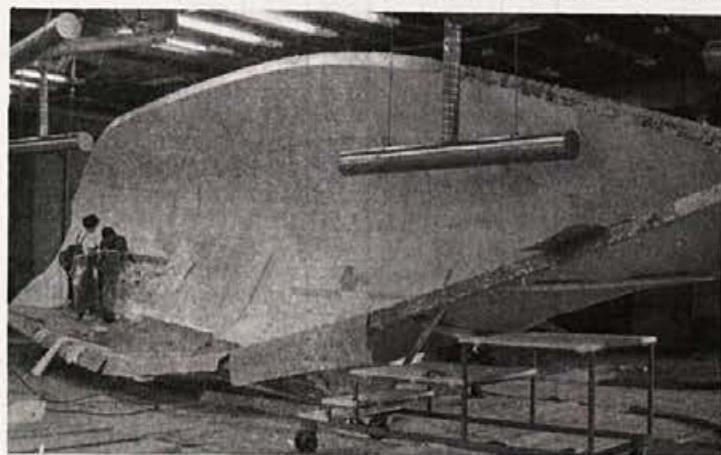
Delo v novi livnici. Veliko laminata je treba položiti za trup E-43
