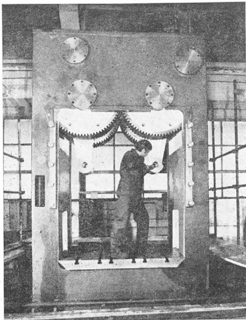
Takšno stiskalnico — velikanko — smo skonstruirali in izdelali v naši železarni
