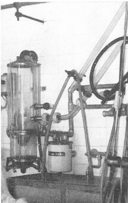
Del molznega stroja na Šratneku
