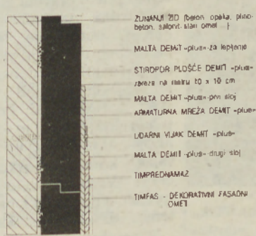
Prerez sistema DEMIT »plus«
