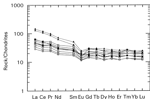
Sl. 7. Na hondrite normalizirane vsebnosti prvin redkih zemelj preiskanih vzorcev predornin s Kozjanskega (poln kvadrat – kislí andezit iz Zagaja, polna trikotnika – dacit iz Trličnega), ter za predornine s Smrekovca (prazni krog, kvadrati, trikotniki).
