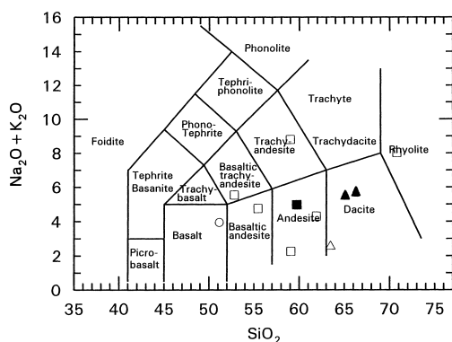
Sl. 6. Diagram vsebnosti alkalij in kremenice (LeBas et al. 1986) za preiskane vzorce predornin s Kozjanskega (poln kvadrat – kislí andezit iz Zagaja, polna trikotnika – dacit iz Trličnega), ter za predornine s Smrekovca (prazni krog, kvadrati, trikotniki).
