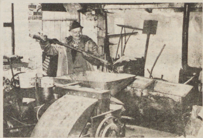
BRIKETIRNIK — Mesarski mojster Ludvik Both je s pomočnikoma izdelal stroj za stiskanje žagovine. Tako je s kurivom gospodinjstvo preskrbljeno, povrh pa je skoraj zastoj. Foto: Š. S.
