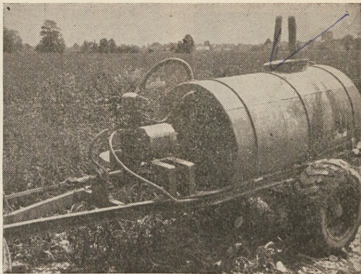
V delavnici na »Osojniku« izdelana traktorska škropilnica. Posnetek: M. Glušič
