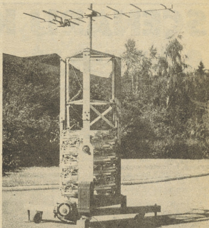
Zložljivi nosilni stolp, ki so ga izdelali mladi strokovnjaki Gorenja Muta
