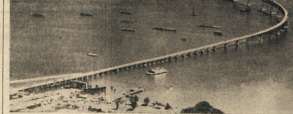
Novi najdaljši jekleni most na svetu čez zaliv Chesapeake v Marylandu (ZDA). Celoten most je dolg 12,36 km; visoki del je dolg 480 m in sloni na dveh 104,4 m visokih opornih stolpih. Cestnice je na tem mestu 55,8 m nad morsko gladino. — Do sedaj so zvezo med obema obalama vzdrževali štiri državne prevozne ladje, voznja pa je trajala 40 minut; sedaj bo trajala le 6 minut.
