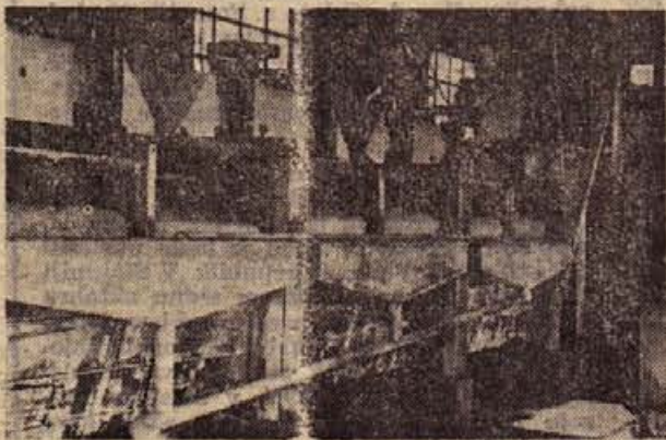
Novo flotacijske naprave v obratu Ravno omogočajo zdaj izvoz najkvalitetnejšega kremenčevega peska, ki ga tovar- ne uporabljajo tudi za proizvodnjo finega stekla in kera- mike
