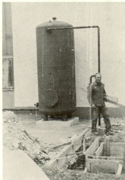
Postavitev in povezava vetrovnika, ki je sestavni del kompresorske postaje
