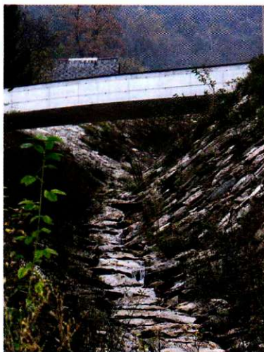
Most sredi Koseča je bil na novo zgrajen leta 2002, vendar je v lokacijskem načrtu predviden nov most, strugo pod njim pa naj bi poglobili za 2 metra. Tako bi bila v primeru plazanja tal pretočnost materiala pod mostom večja in vas ne bi bila tako ogrožena.
