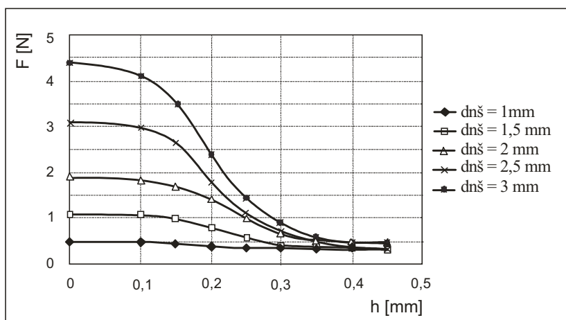
Sl. 12. Potek odvisnosti sile F od odmika odbojne plošče in premera nastavljive šobe Fig. 12. Force, F , versus flapper displacement for various adjustable nozzle diameters
