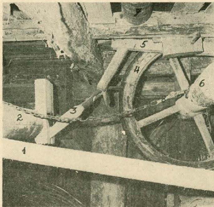
Prenosni pogonski mehanizem pod žagalnico navadne potočne žage venecijanke
