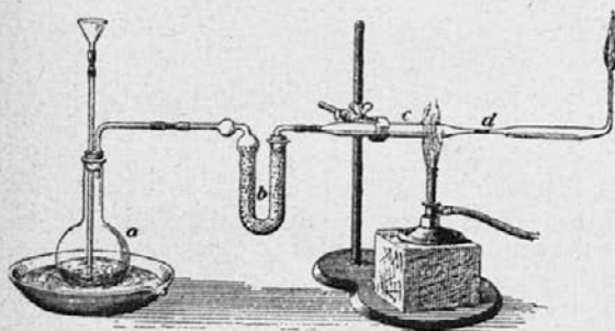
Sl. 1. Mitscherlichova aparatura za dokazovanje fosfora.
