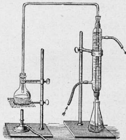
Sl. 2. Aparatura za dokazovanje arzena po Marshovi metodi.
