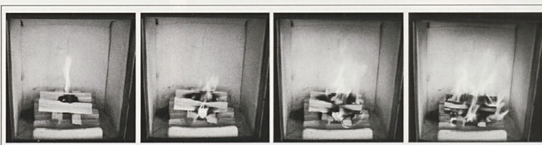
Prikaz primerne zakuritve (Vir: TFZ Bayern)
