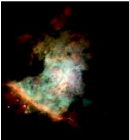
Velika orionova meglica M 42
