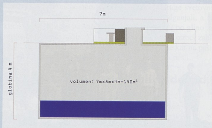
Zgoraj: Prerez vodnjaka
