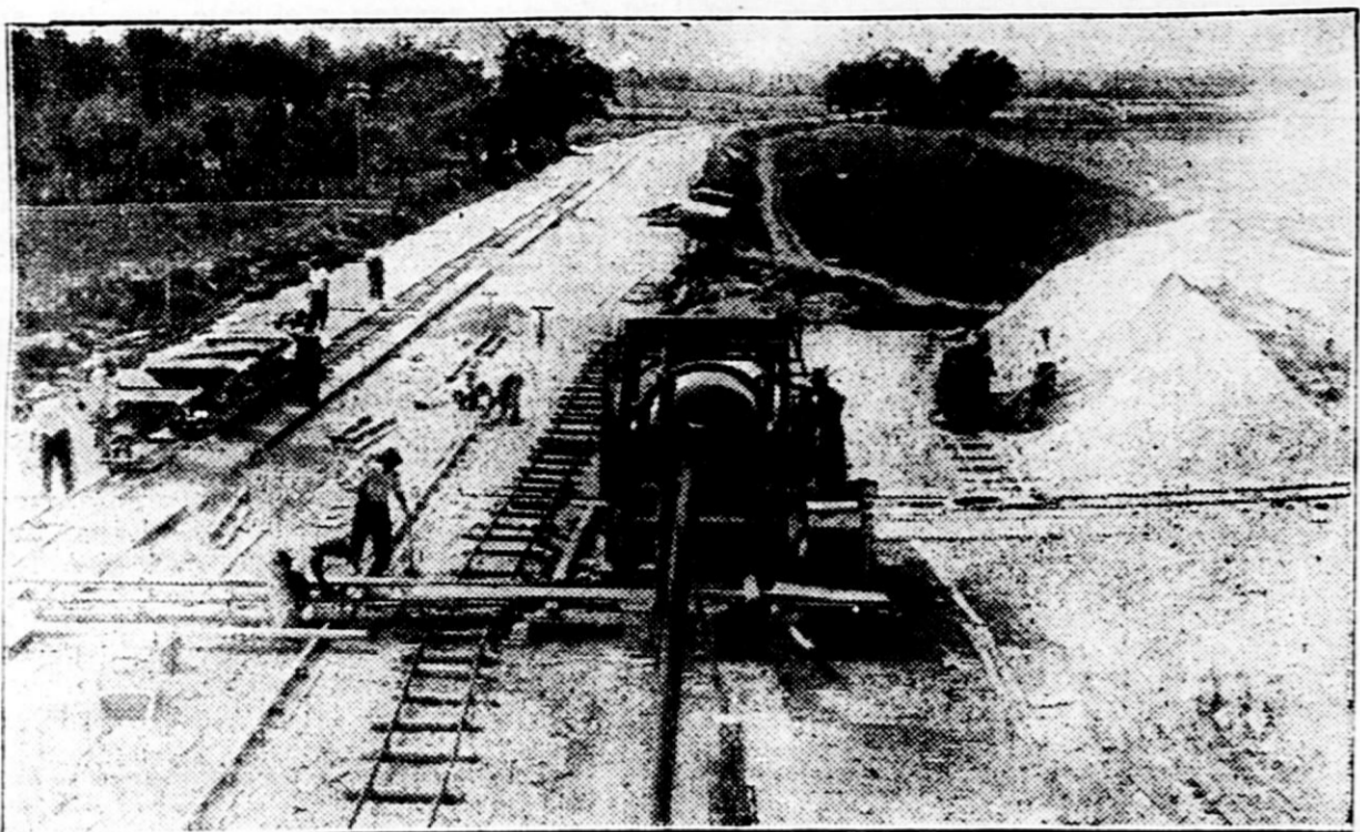
Del že zbetoniranega cestnišča (brez robnih trakov) na odseku Kranj — Naklo
