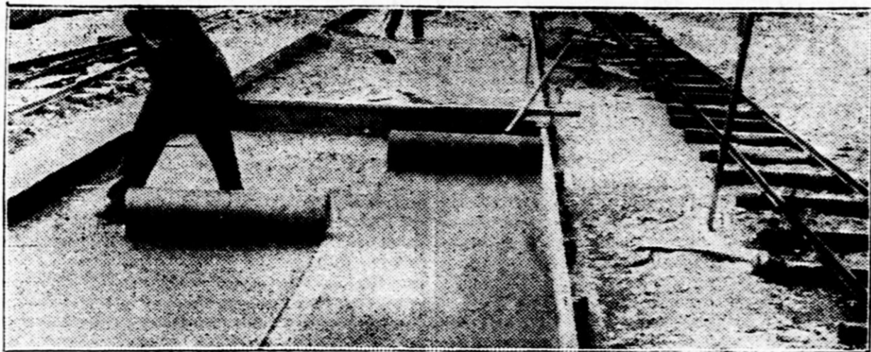
Polaganje impregiranega papirja, na katerega nato nasujejo betonsko mešanico
