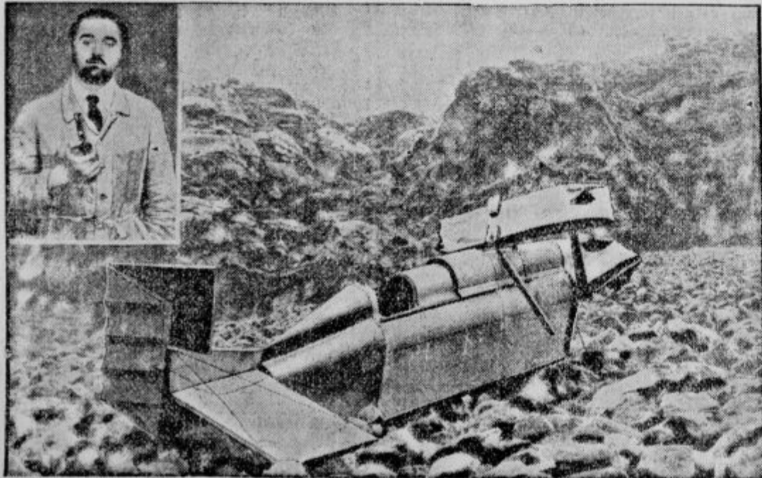
Prostovoljen padec s letalom. Francoski izumitelj Sauvant je napravil posebno letalo, katerega trup je zgrajen na poseben način. Po zatrevljanju izumitelja nudi tako letalo popolno sigurnost za življenje potnikov tudi v slučaju nevarnih padcev z višin. Ker mu policijske oblasti niso dovolile, da bi napravil poskuse v Parizu, je te dni izumitelj s svojim letalom odplul v oddaljeno provinco in se pri kraju Escagnolles strmoglavil z velike višine na skalnato hribovje. Kakor je videti, je bilo letalo zelo poškodovano, trup je ostal popolnoma ohranjen in tudi drzni letalec je ostal živ in zdrav.
