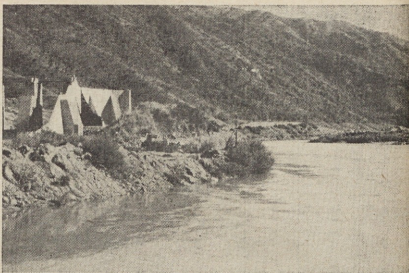
Reka Great Ruaha, kjer je bil pozneje zgrajen jez za elektrarno. Na sliki se vidijo že temelji segmentnih zapornic.
