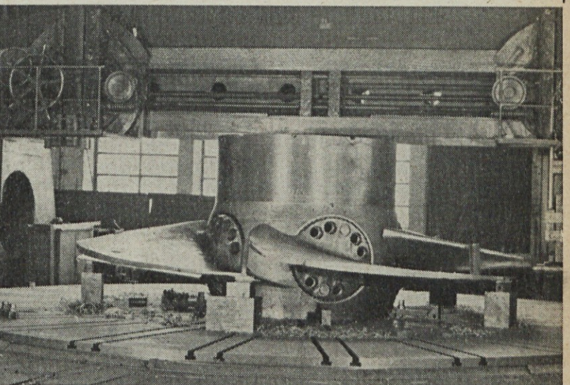
Tekač za HE Varaždin, ko je bil še na obdelovalnem stroju
