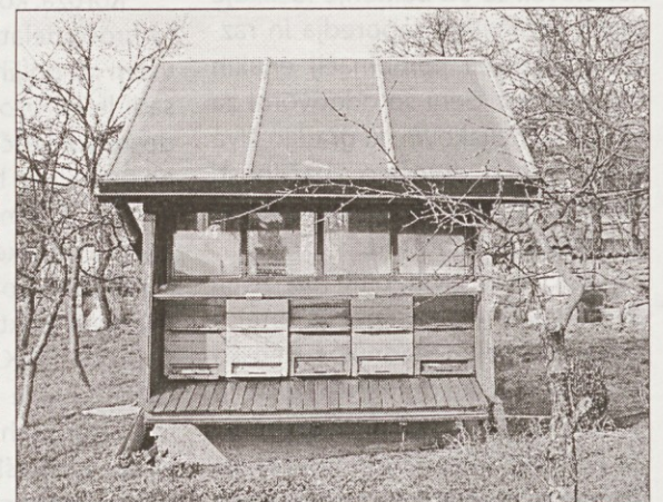
Samogradnja sprejemnikov sončne energije cca 8m2 in postavitve na čebelnjaku, cevi speljane v kotlovnico v dolžini cca 70m, boiler 300 l Frlež Janko iz Jasena.
