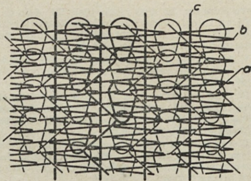
Shema vezave pri prešitem blagu
