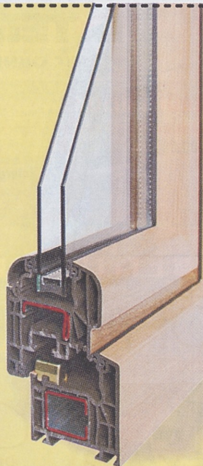
PVC okno - CT 70, 5 komor
