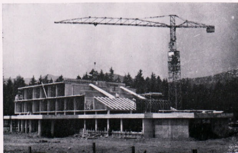
Na hotelu v Zrečah so pričeli polagati strešno konstrukcijo.
