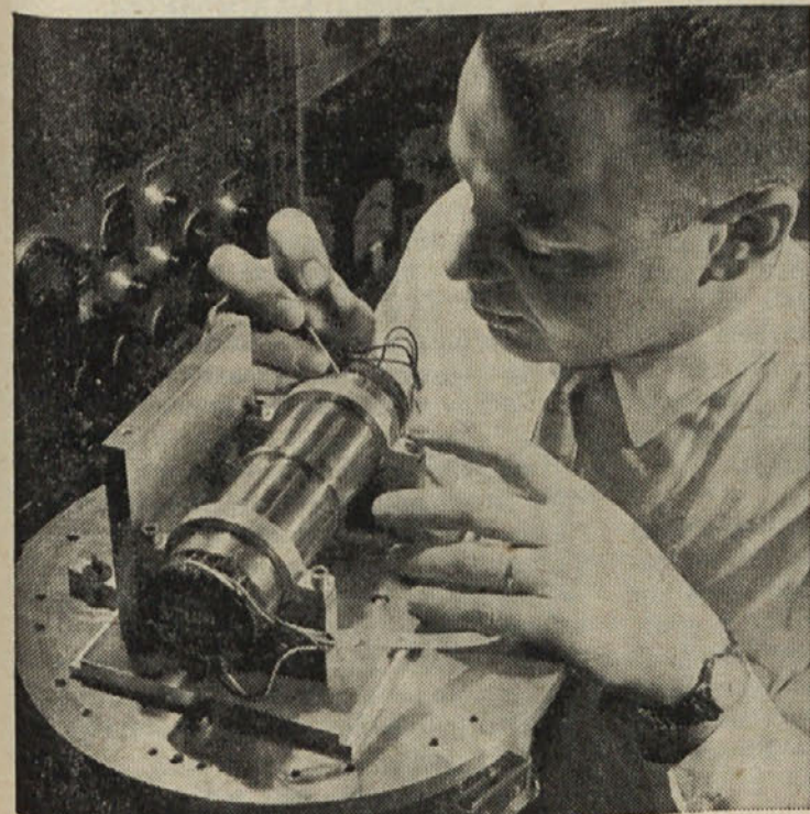
Na sliki vidimo zboljšani krožni kompas, ki ga preskušajo na Long Islandu v Ameriki. Namesto vrtečih kolesc uporabljajo vrtečo tekočino. Če se bo ta naprava obnesla, jo bodo pozneje uporabili za stabilizacijo postaj v vesolju.
