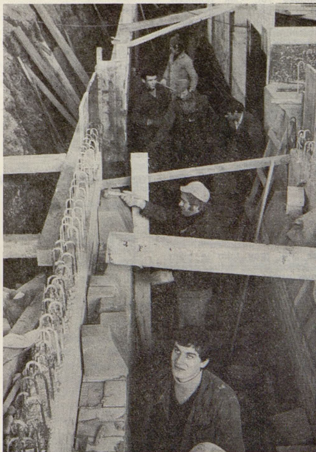
Obzidava kanala
