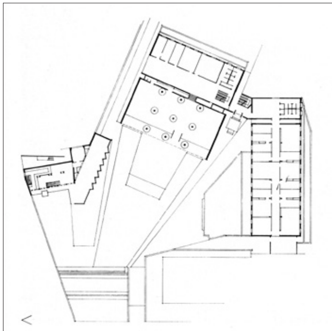
Tloris pritličja kompleksa MO Kranj
