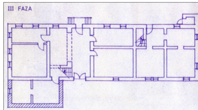
Tloris pritličja z zahodnim in severnim prizidkom, hrani ZVKDS, OE Kranj.
