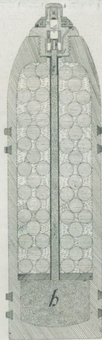
Šrapnel v prerezu.
