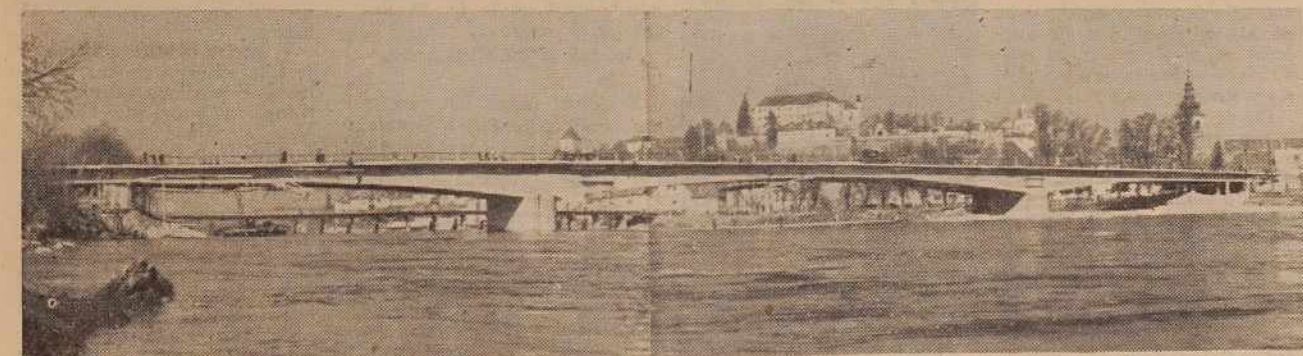
Minulo nedeljo so predali v Ptuj prometu nov sodoben most čez reko Dravo. (na sliki) Most, ki ga je zgradilo po lastnem projektu podjetje »Tehnogradnja« iz prednapetega betona na brezoderni način (10 m široko vozišče), nima le lokalnega pomena, ampak je hkrati tudi najlažji prehod in najkrajša pot iz Panonije v alpski in kraški svet ter dalje v Italijo.
