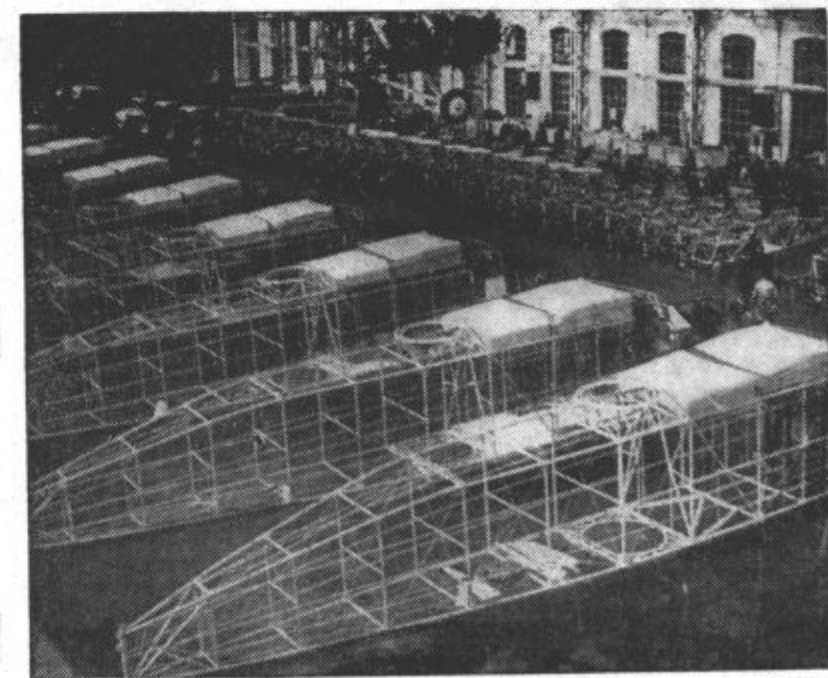
ITALIJA SE OBOROŽUJE. Pogled v veliko delavnico za letala v okolico Rima, kjer izdelujejo lovška letala in aeroplance za bombardiranje
