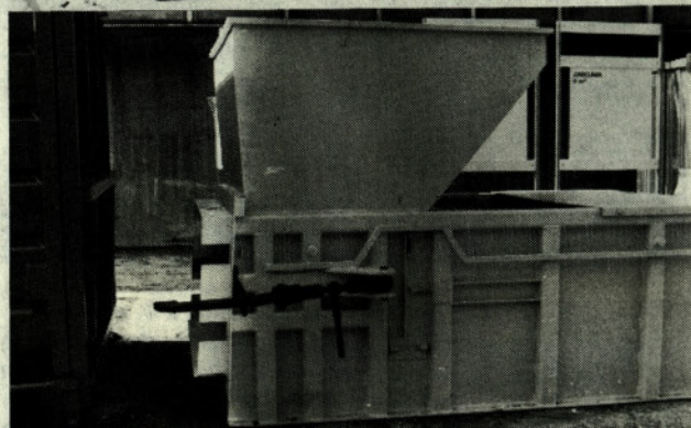
Kotalni prekucnik – rol kiper smo sicer v preteklosti že predstavili, vendar smo ga medtem dodatno opremili, izpopolnili oz. dopolnili z stacionarno stiskalno napravo, s čimer se je njegova uporabnost in izkoriščenost še povečala.
